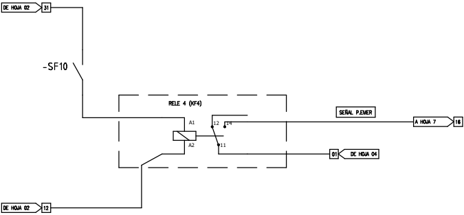
Señal Parada de Emergencia Para 3.3v-5v-12v-24v
