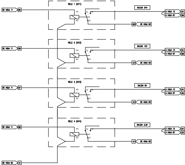
Conexionado Relevos de salidas 24-12-5-3.3 Voltios (pulsos)
