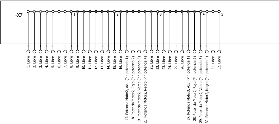
-CONECTOR_2 (POTENCIA MOTORES)
