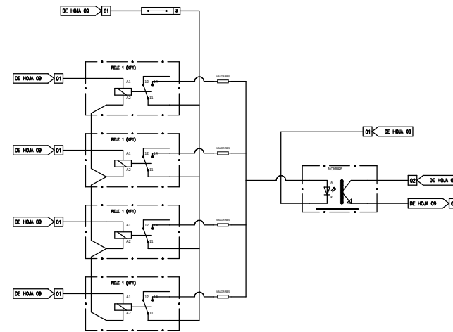
Conexionado de Pulsos (DIR+ DIR- EJE X)
