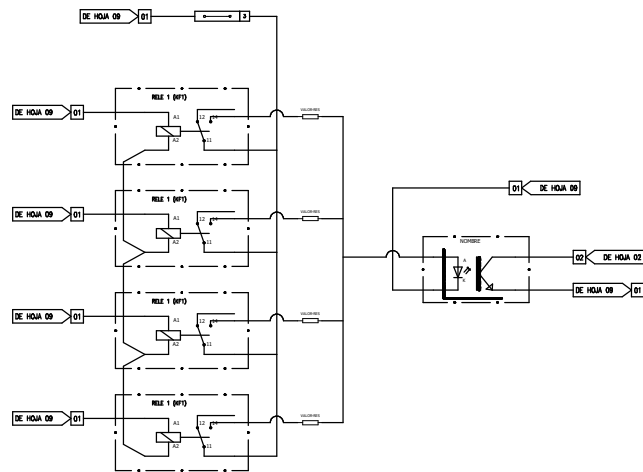
Conexionado de Pulsos (EN+ EN- EJE X)
