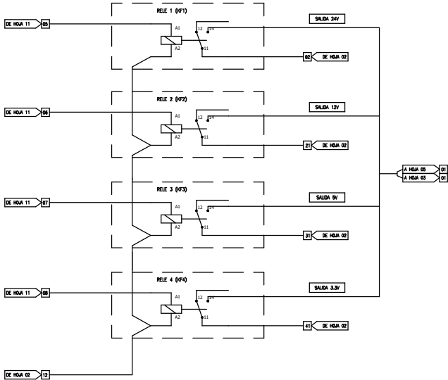
Conexionado Relevos de salidas 24-12-5-3.3 Voltios (pulsos)
