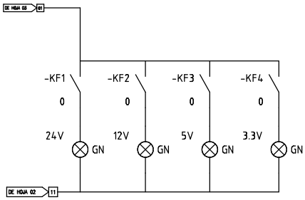
Conexion Pilotos Fuentes
