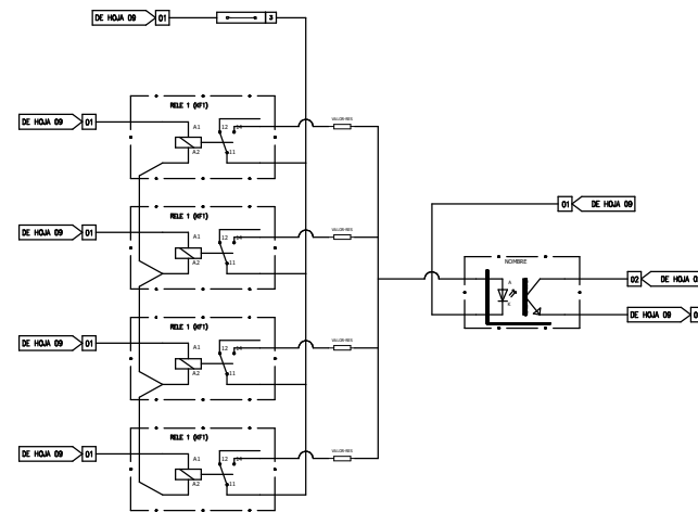
Conexionado de Pulsos (EN+ EN- EJE Y)
