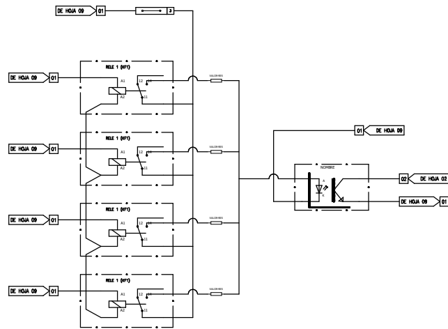
Conexionado de Pulsos (EN+ EN- EJE Z)
